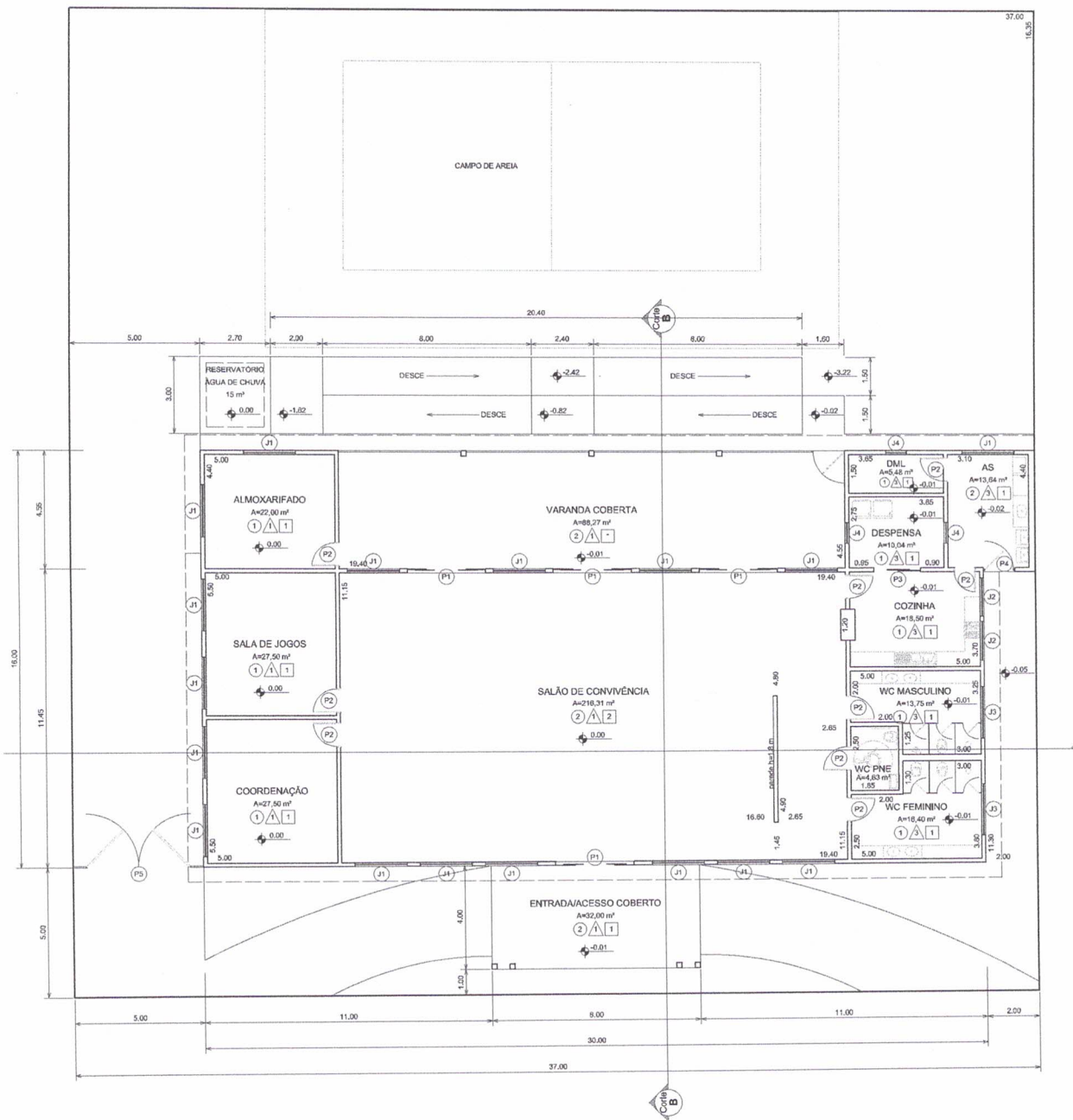
PLANTA BAIXA ESCALA 1:100
